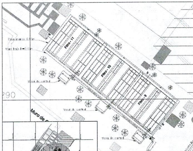
Ilustración 2 Unidades de filtración que se requiere intervenir.
