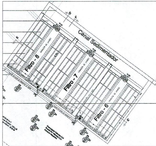
Ilustración 1 Ejecución de la fase 1 de la optimización Filtro 6, 7 y 8 , contrato 066-21
