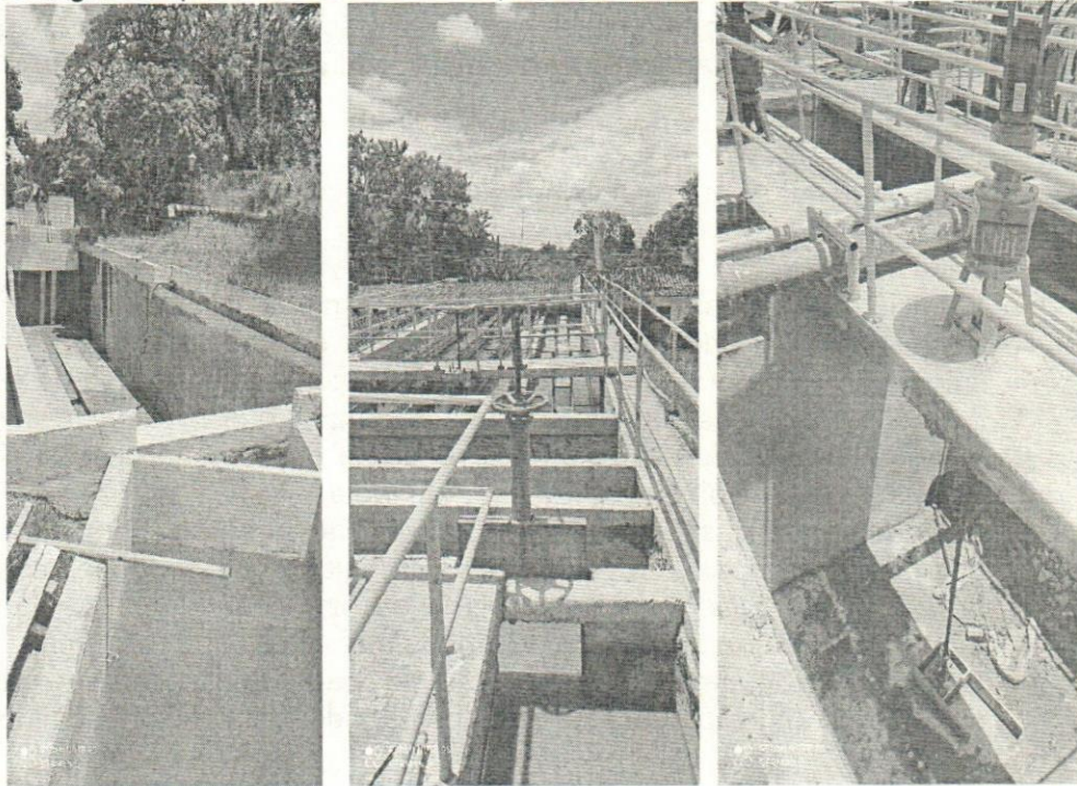
Fuente. Acuavalle Obras de optimización PTAP Andalucía 07/03/2022
