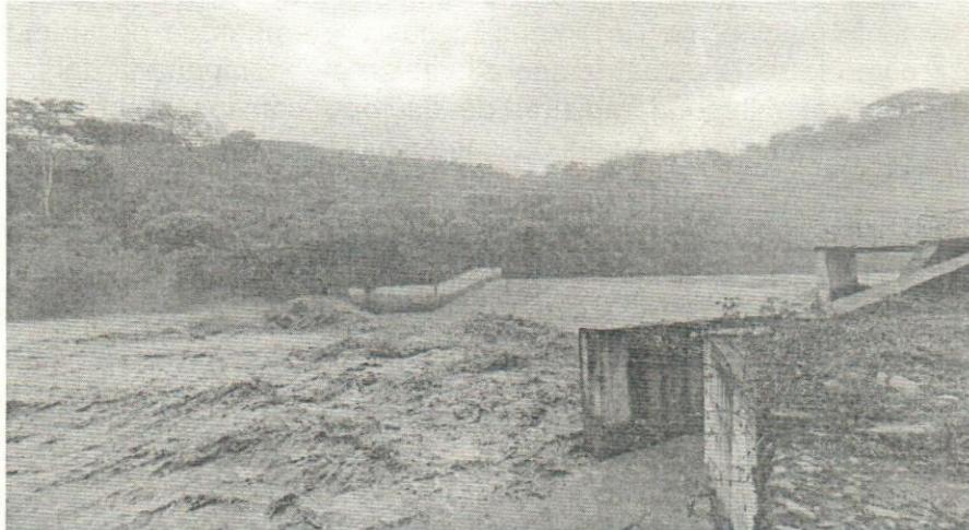
Foto 1. Bocatoma Voladeros. 07/03/2022
