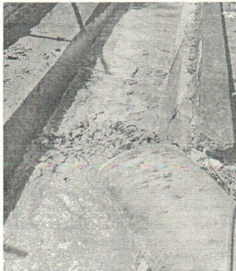
Foto 5. Llegada agua cruda PTAP ANDALUCIA. 07/03/2022. 10:45 AM
